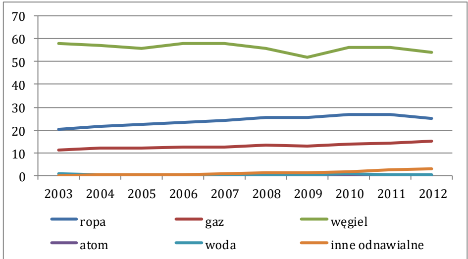
Wykres 2. Źródła energii w Polsce w latach 2003-2012 [w Mtoe].
